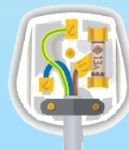
wires
